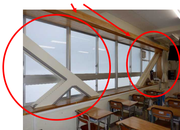
耐震補強（3の8教室）
